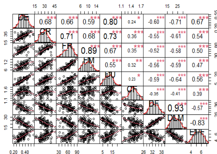
Figura 2: Matriz de correlação de Pearson entre as propriedades da madeira de Schefflera morototoni. DE: Densidade básica; CR: Resistência à compressão paralela; FR: Resistência à flexão estática; FM: Módulo de elasticidade na flexão estática; DU: Dureza dinâmica; CF: Comprimento de fibra; DF: Diâmetro da fibra; DLM: Diâmetro do lume da fibra; EPF: Espessura da parede da fibra. Códigos do valor de p de significância: 0 ‘***’; 0,001 ‘**’; 0,01 ‘*’; 0,05.
